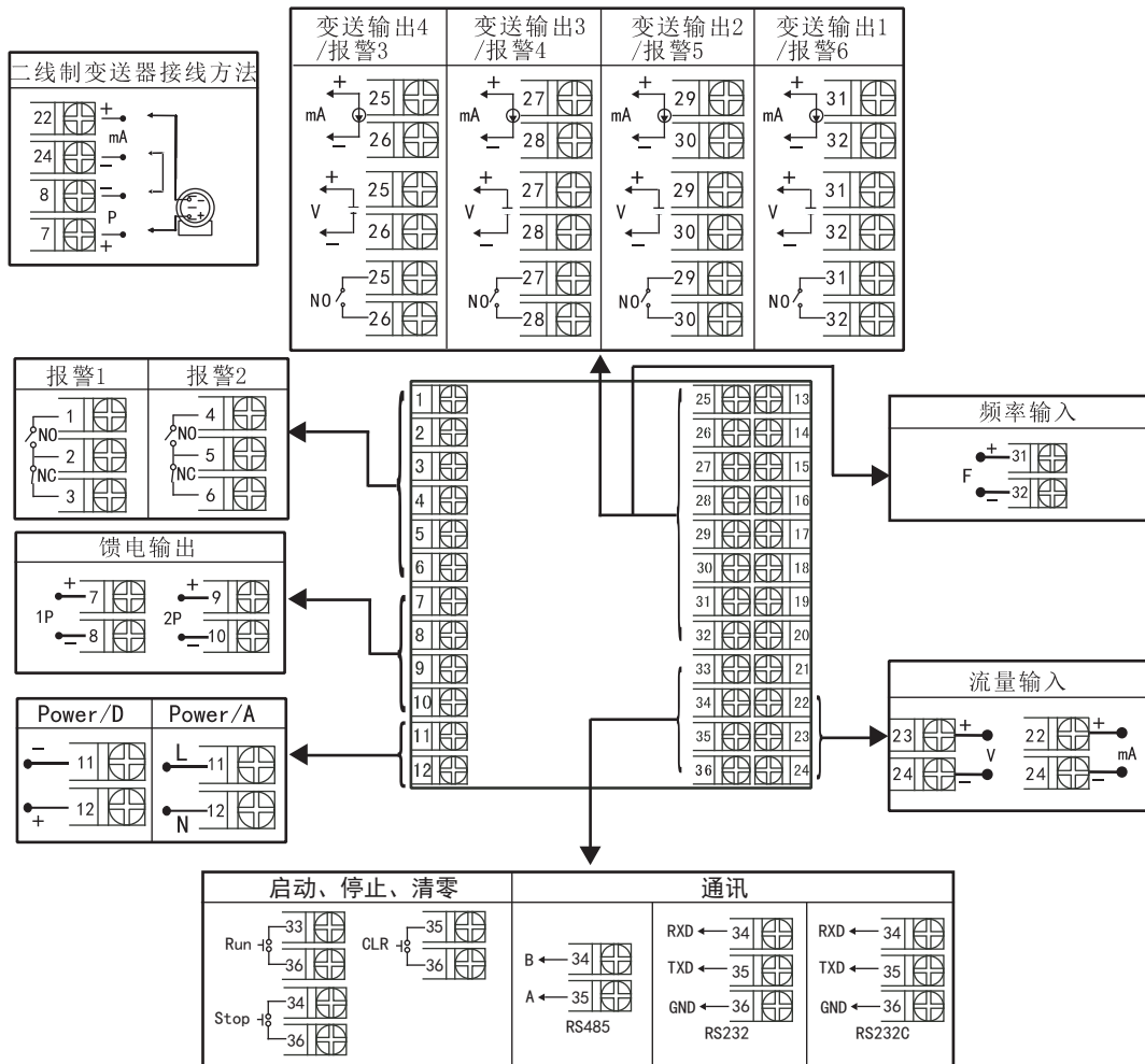
NHR-7601/7601R系列接线图
